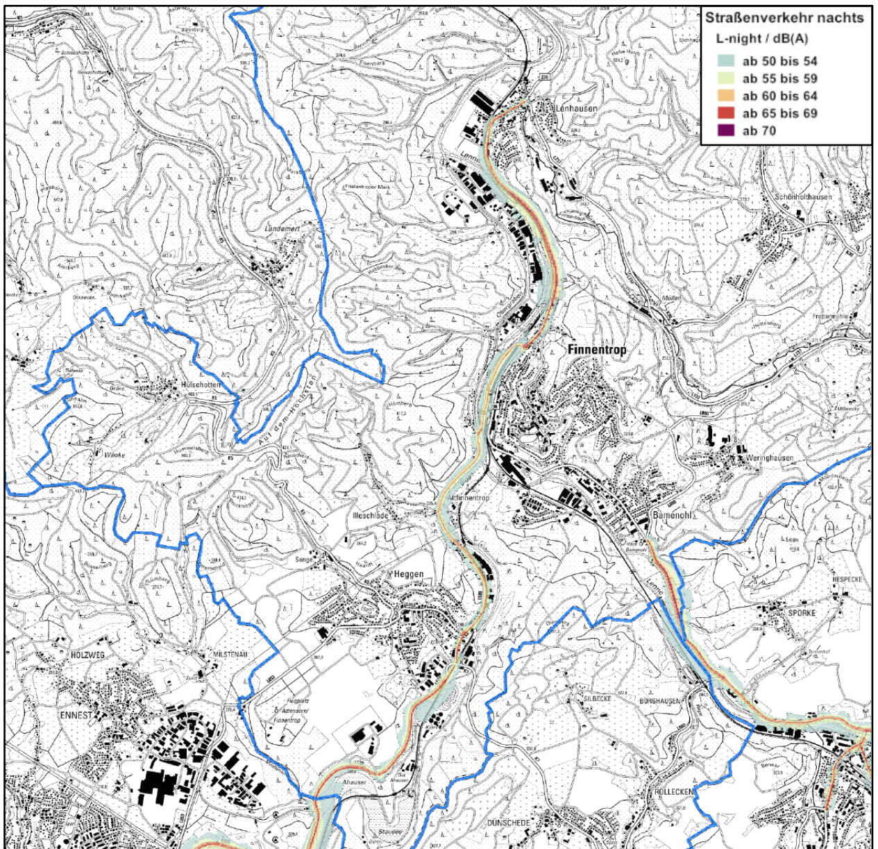
Karte 2: Isophonenkarte Nacht L_{night} Gemeindegebiet Finnentrop, genordet, ohne Maßstab (Auszug aus Anlage 3)
