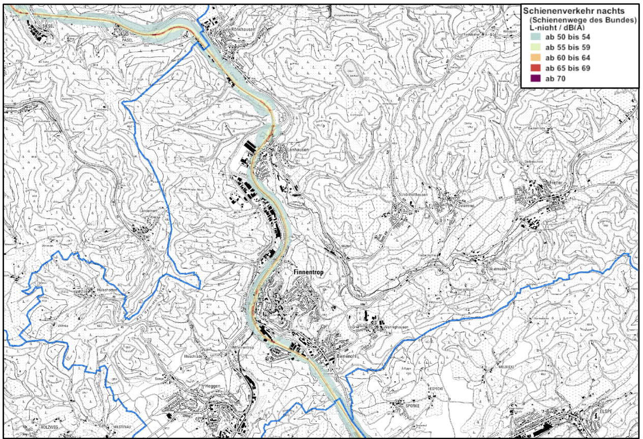
Karte 4: Isophonenkarte Schiene Nacht L_{night} , genordet, ohne Maßstab (Auszug aus Anlage 5)
